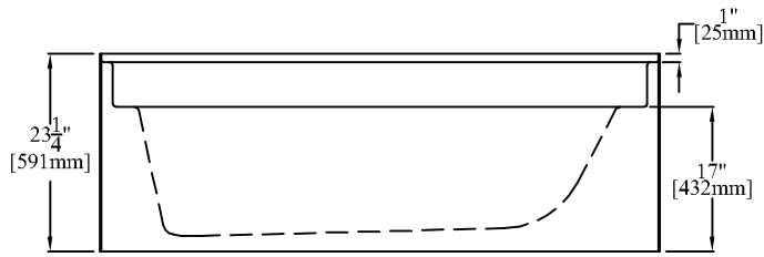
ELEVATION
