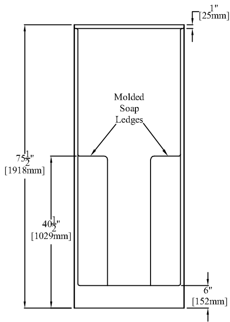
ELEVATION
