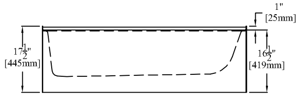
ELEVATION
