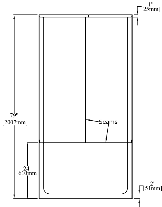
ELEVATION
