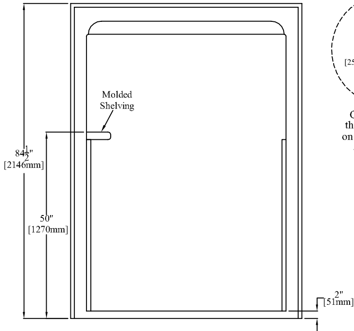
ELEVATION
