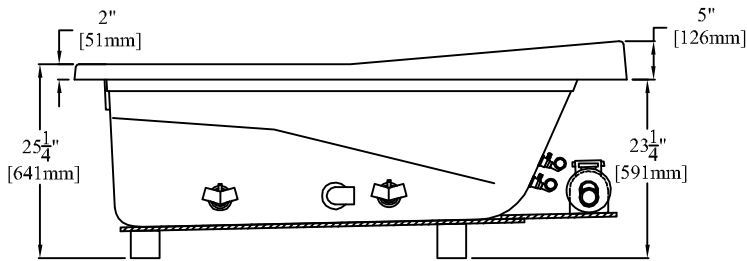
ELEVATION
