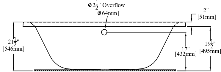
ELEVATION
