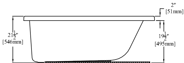
ELEVATION
