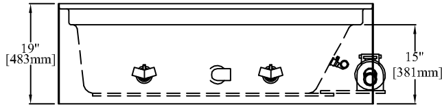
ELEVATION
