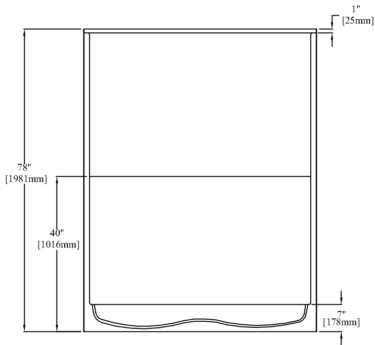
ELEVATION
