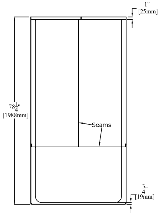
ELEVATION
